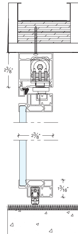
SINGLE GLAZED PIVOT DOOR WITH DROP SEAL AND CLOSER PORTE PIVOT EN VERRE SIMPLE AVEC SEUIL DE PORTE TOMBANT ET FERMOIR
