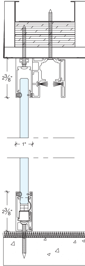
SINGLE GLAZED FRAMED SLIDING DOOR IN CLOSED POSITION PORTE COULISSANTE ENCADRE EN VERRE SIMPLE EN POSITION FERMÉE
