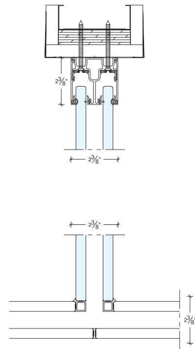
DOUBLE GLAZED T CONDITION RETOUR EN T EN VERRE DOUBLE
