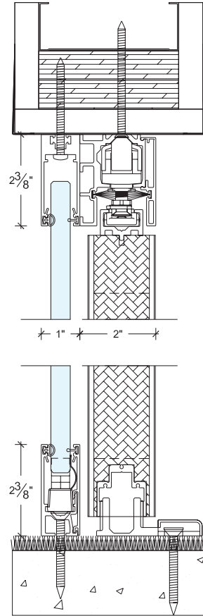
WOOD SLIDING DOOR IN THE OPEN POSITION PORTE COULISSANTE EN BOIS EN POSITION OUVERTE
