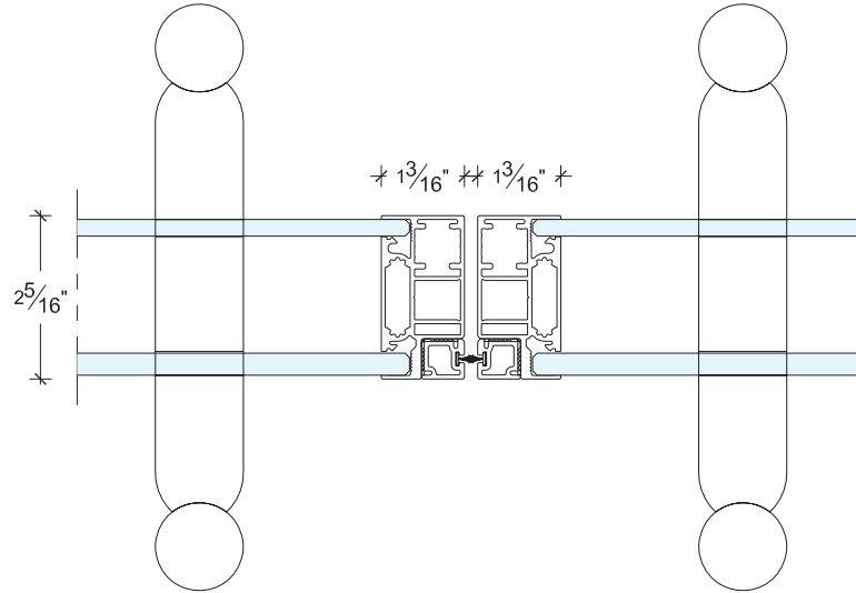
DOUBLE GLAZED DOUBLE LEAF DOOR WITH LADDER PULL PORTE DEUX VANTAUX EN VERRE DOUBLE AVEC POIGNÉE TUBULAIRE
