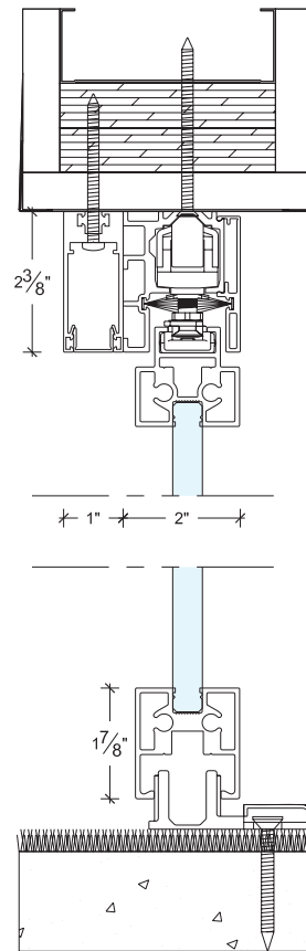
SINGLE GLAZED FIXED GLASS SIDELIGHT VEILLEUSE FIXE EN VERRE SIMPLE
