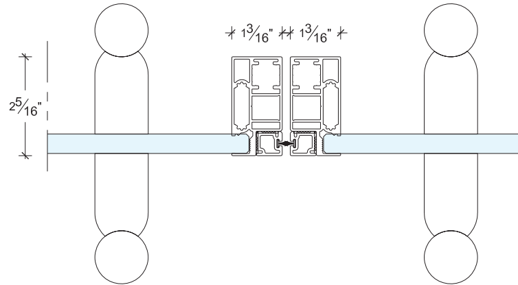
SINGLE GLAZED DOUBLE LEAF DOOR WITH LADDER PULL PORTE DEUX VANTAUX EN VERRE SIMPLE AVEC POIGNEE TUBULAIRE
