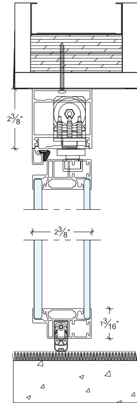
DOUBLE GLAZED PIVOT DOOR WITH DROP SEAL AND CLOSER PORTE PIVOT EN VERRE DOUBLE AVEC SEUIL DE PORTE TOMBANT ET FERMOIR
