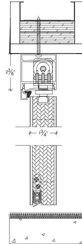
WOODEN PIVOT DOOR WITH DROP SEAL PORTE PIVOT EN BOIS AVEC SEUIL DE PORTE TOMBANT
