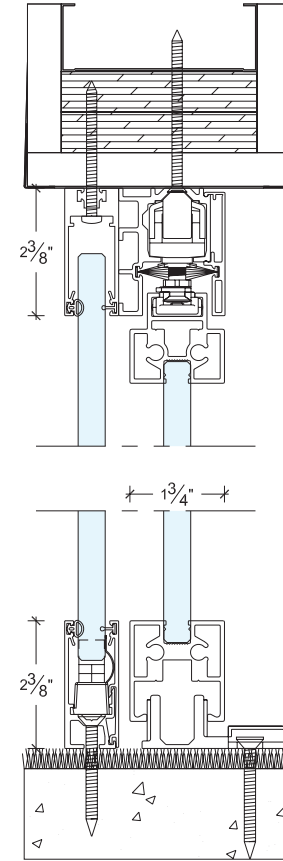
SINGLE GLAZED FRAMED SLIDING DOOR IN OPEN POSITION PORTE COULISSANTE ENCADRE EN VERRE SIMPLE EN POSITION OUVERTE
