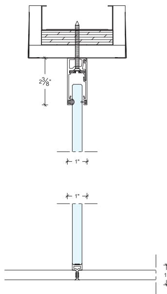
SINGLE GLAZED T CONDITION RETOUR EN T EN VERRE SIMPLE
