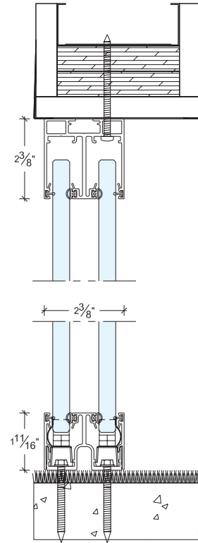
TOP AND BOTTOM PROFILE IN DOUBLE GLAZE ON A BULKHEAD CEILING PROFIL SUPÉRIEUR ET INFÉRIEUR EN VERRE DOUBLE SUR RETOMBÉE DE PLAFOND
