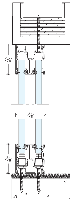
TOP AND BOTTOM PROFILE IN DOUBLE GLAZE ON A BULKHEAD CEILING PROFIL SUPÉRIEUR ET INFÉRIEUR EN VERRE DOUBLE SUR RETOMBÉE DE PLAFOND
