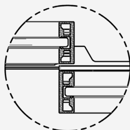
Verre simple en position fermée
