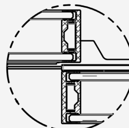
Verre double en position fermée
