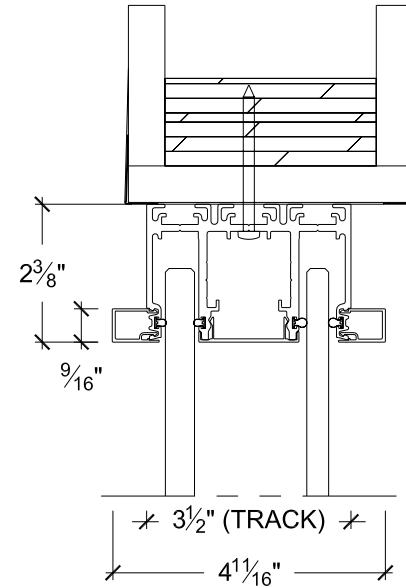
Top profile with double 1/2" and 3/8" glass on bulkhead ceiling Profil supérieur avec verre double de 1/2 po et 3/8 po sur retombée de plafond
